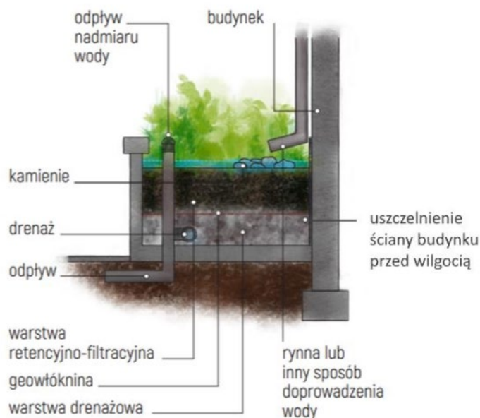
Rysunek 37. Schemat ogrodu deszczowego (źródło: www.budzet.krakow.pl )
