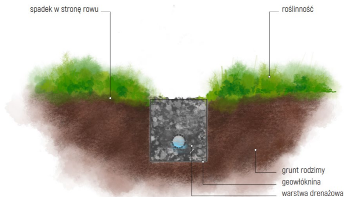
Rysunek 36. Schemat rowu infiltracyjnego (źródło: www.budzet.krakow.pl )
