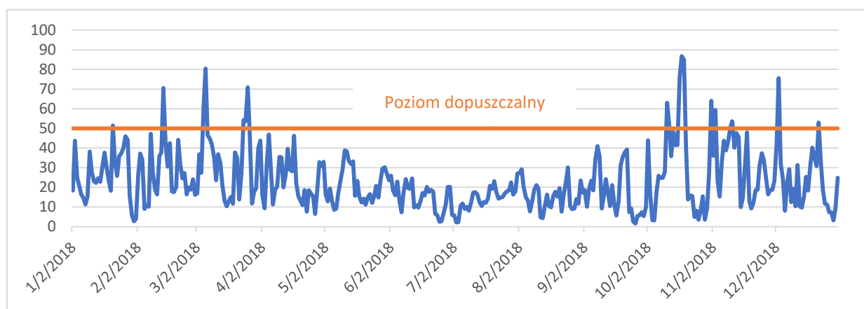
Wykres 14 Poziom pyłu zawieszonego PM10 w Ełku w 2018 r. (źródło: www.powietrze.gios.gov.pl ).
