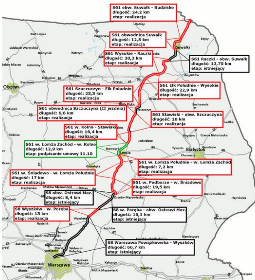
Rysunek 11 Trasa S61 (Via Baltica) w podziale na poszczególne odcinki (źródło: GDDKiA).
