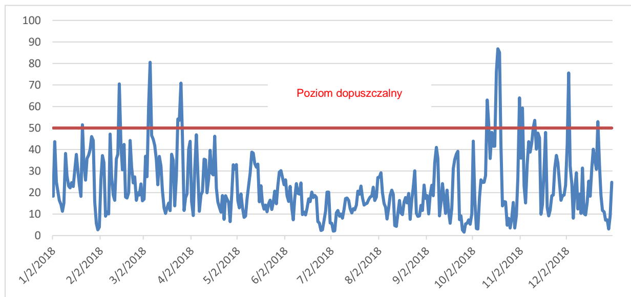
Wykres 22 Poziom pyłu zawieszonego PM10 w Ełku w 2018 r. ( www.powietrze.gios.gov.pl ).
