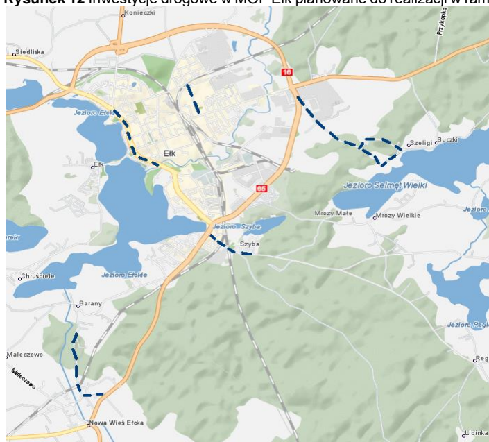
Rysunek 12 Inwestycje drogowe w MOF Ełk planowane do realizacji w ramach ZIT – priorytet inwestycyjny 4e (lista indykatywna).
