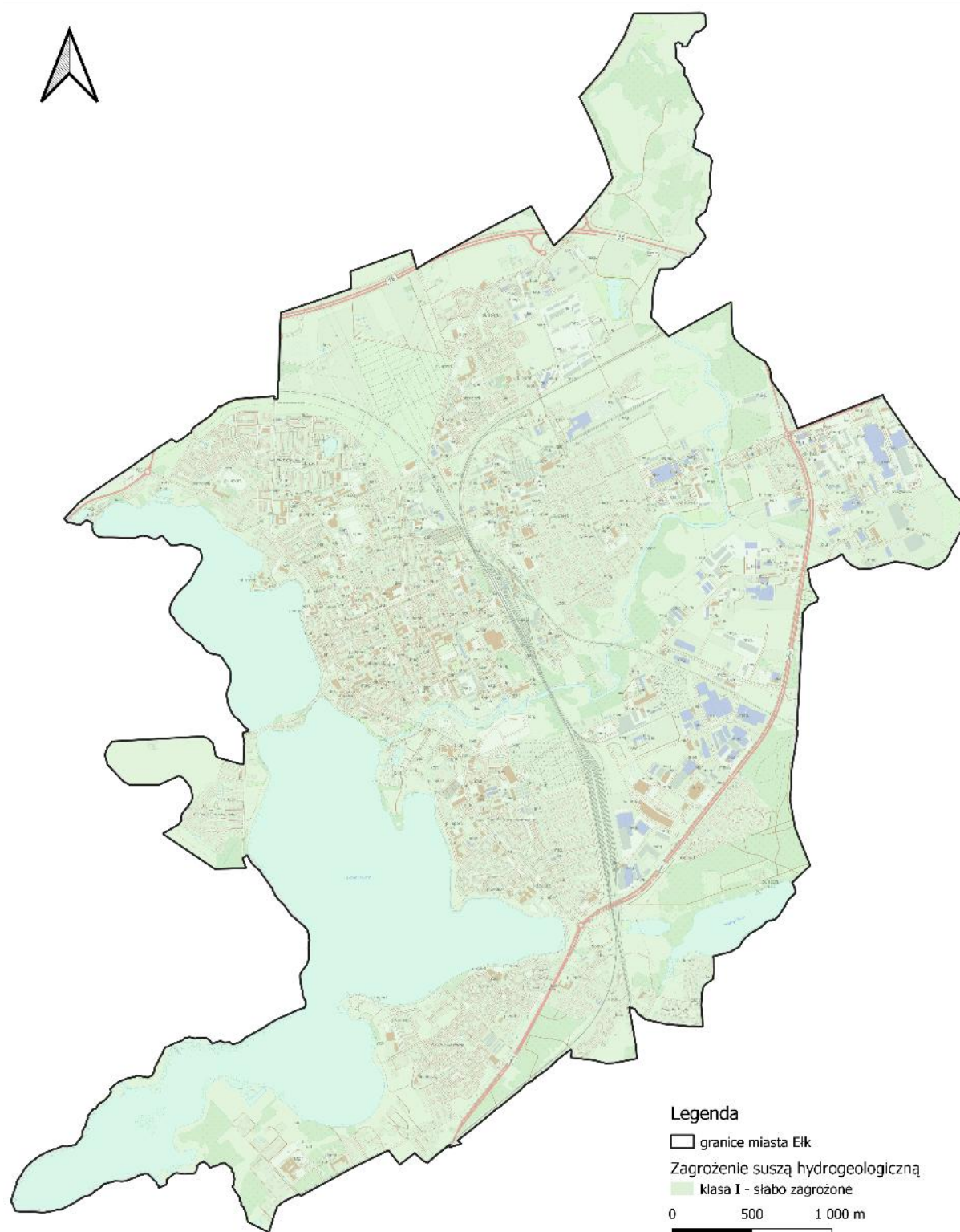
Rysunek 27. Zagrozenie suszą hydrogeologiczną na terenie miasta Elku źródło: opracowanie własne na podstawie strony internetowej: www.wody.isok.gov.pl
